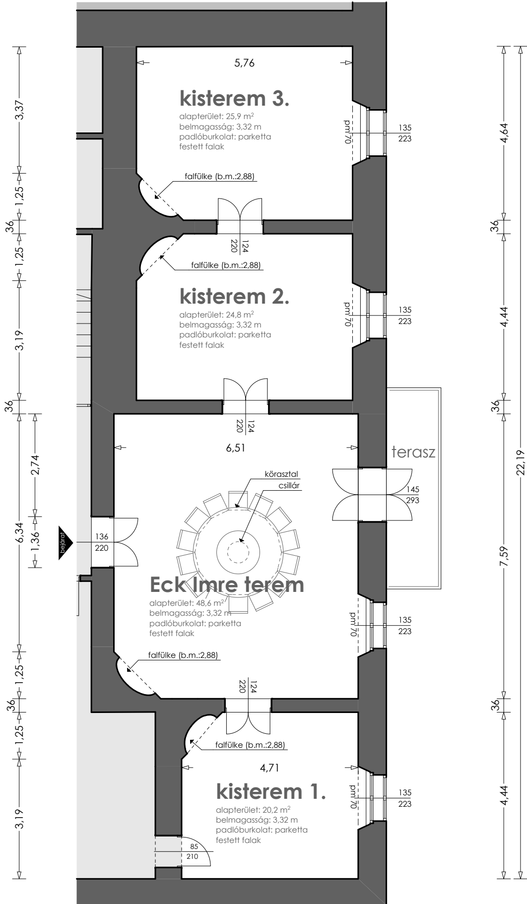
Pécs, Művészetek Háza I.Emelet -Eck Imre terem- M1:100
